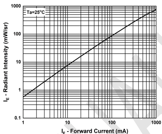
相对辐射功率与正向电流的关系
