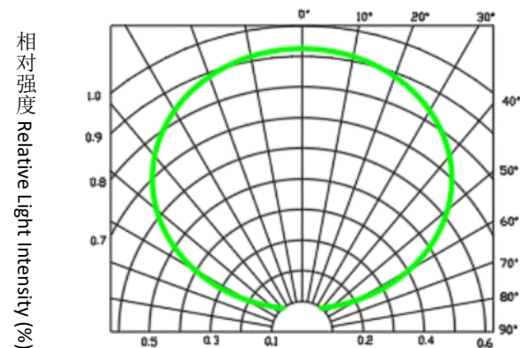
相对光强度与角位移的关系 Relative Light Intensity vs. Angular Displacement
