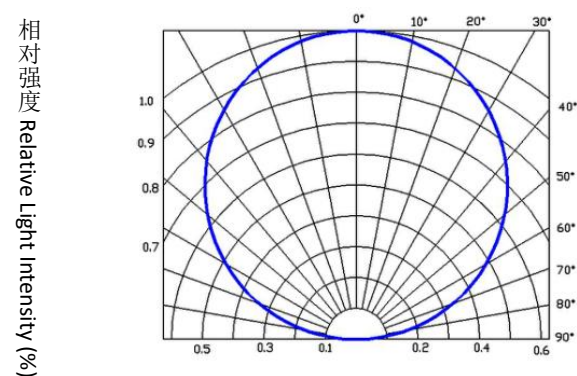
相对光强度与角位移的关系 Relative Light Intensity vs. Angular Displacement
