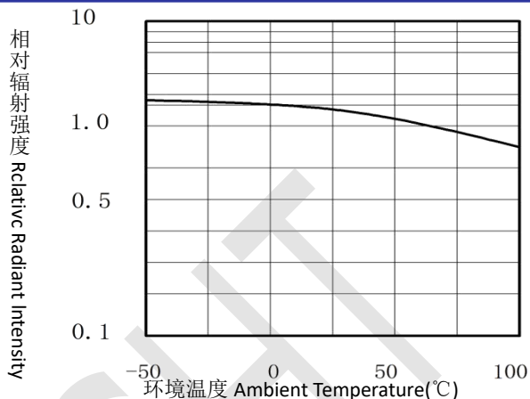
输出特性 Output Characteristics
