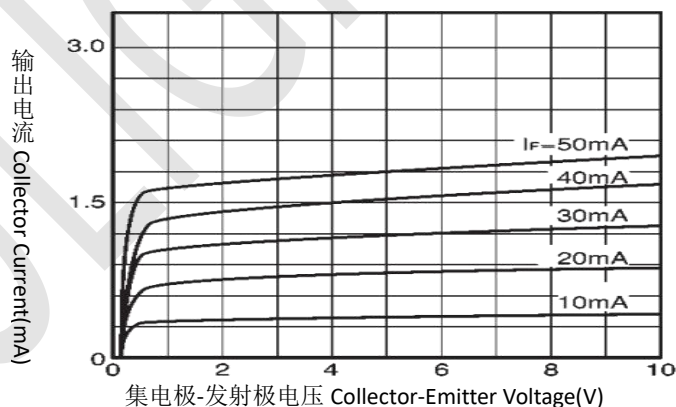
输出特性 Output Characteristics
